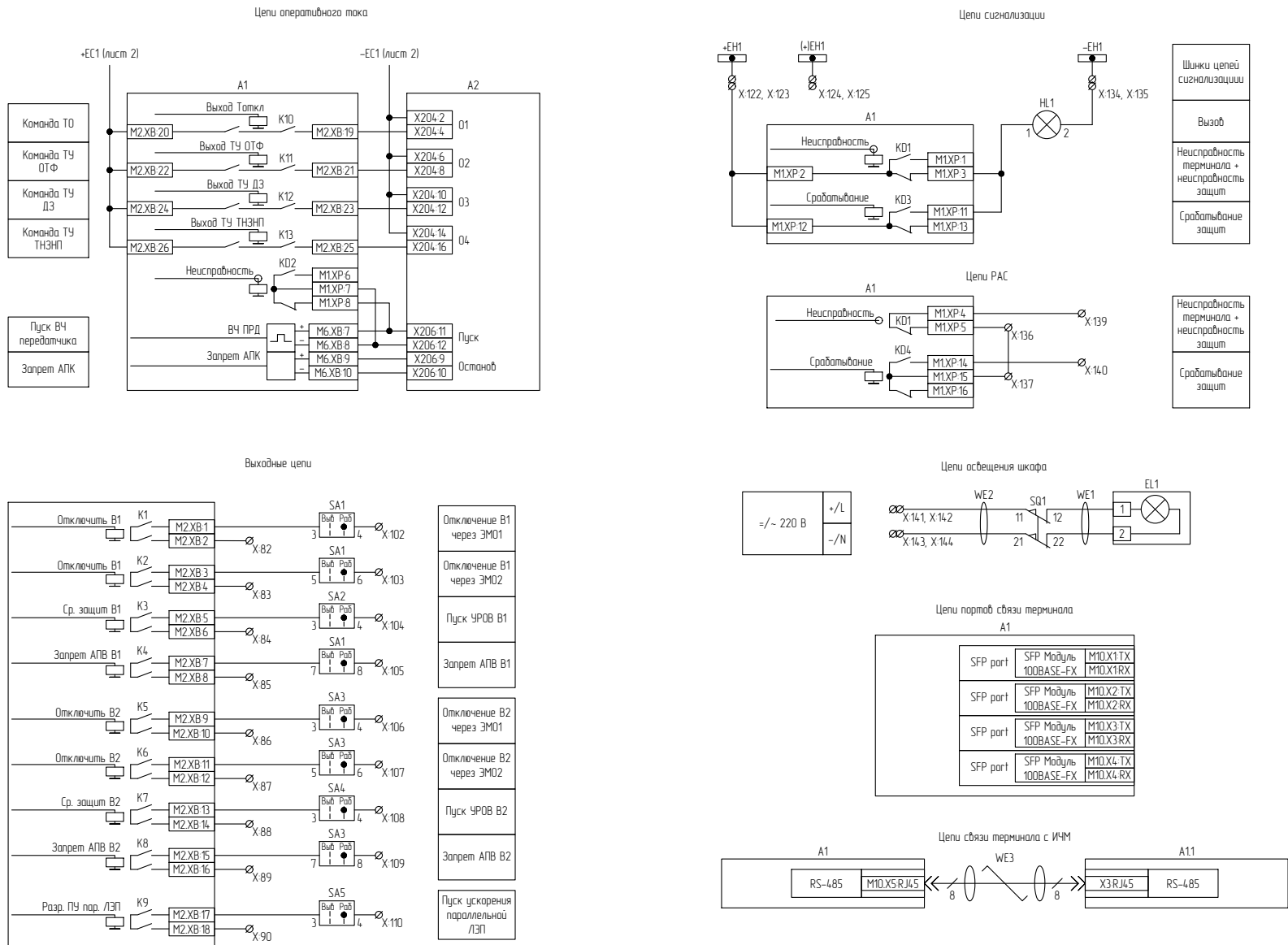
Рисунок В.3 – Схема электрическая принципиальная (часть 3)
