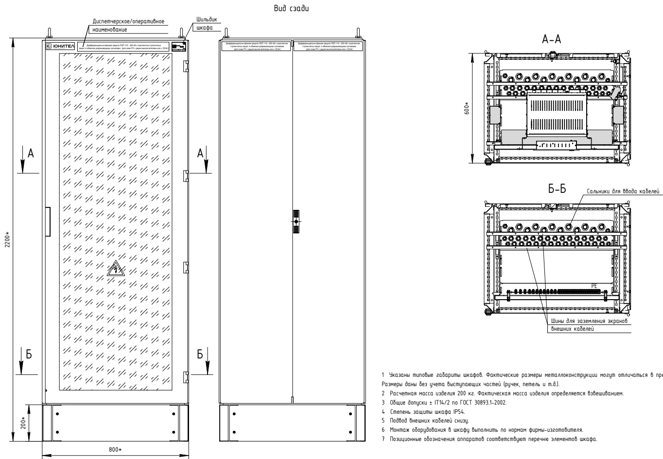
Рисунок Б.1 – Чертеж общего вида (часть 1)
