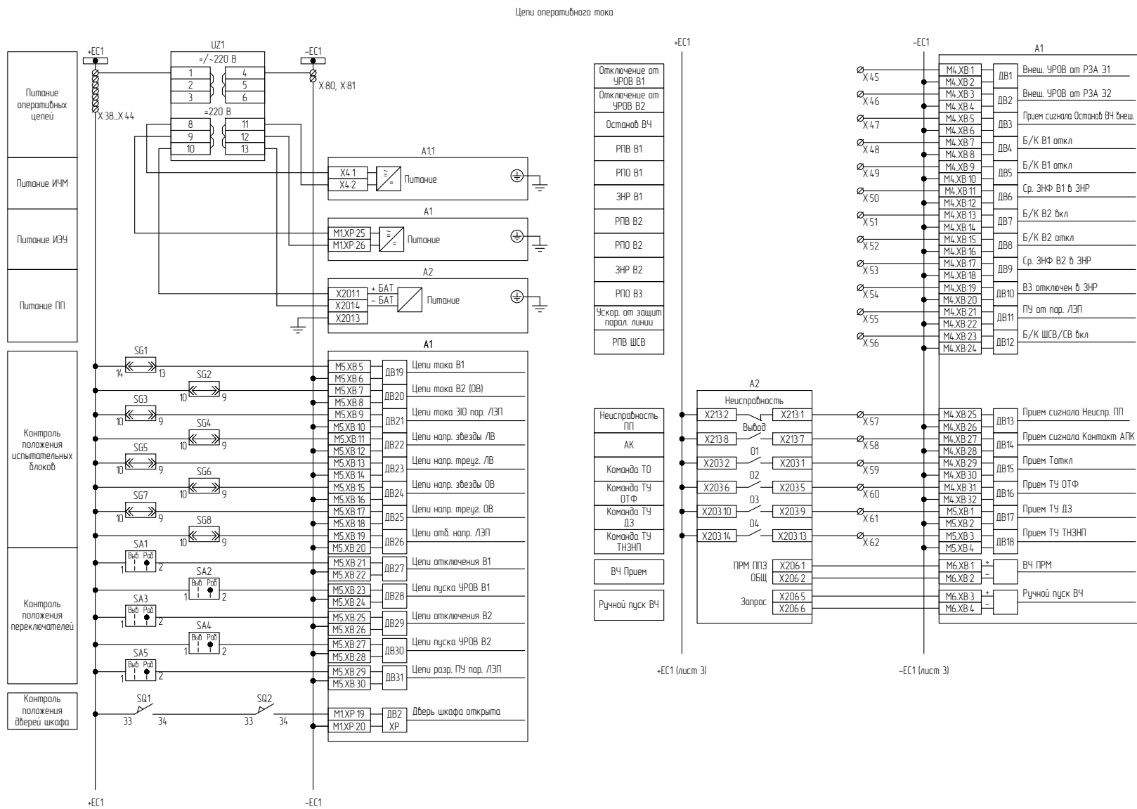
Рисунок В.2 – Схема электрическая принципиальная (часть 2)
